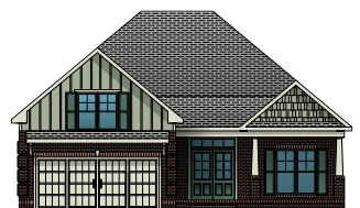
ELEVATION B
